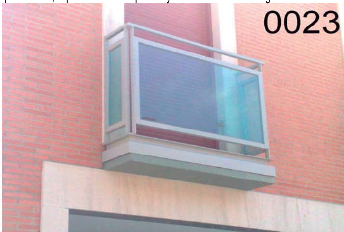
BB-0023: Balcón de acero macizo, tubos y lunas laminaras, verticales de pletina 40*8 mm., cercos ajunquillados de 40*30 mm., pasamanos, imprimacion "wash primer" y lacado al horno gris.
